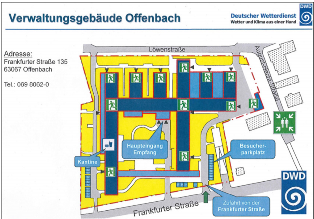
Gebäudeplan
